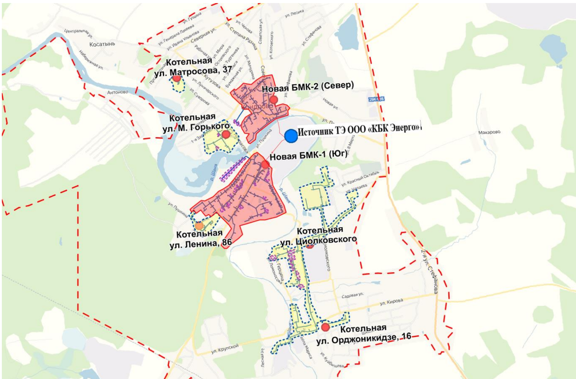
Рисунок 2.1.2-1 - Перспективные зоны действия котельных
