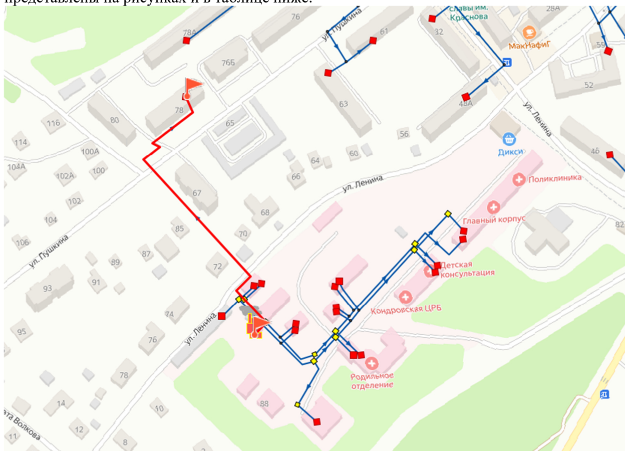
Рисунок 7 - Путь движения теплоносителя от источника тепловой энергии до конечного потребителя, в зоне действия котельной ул. Ленина, 86
