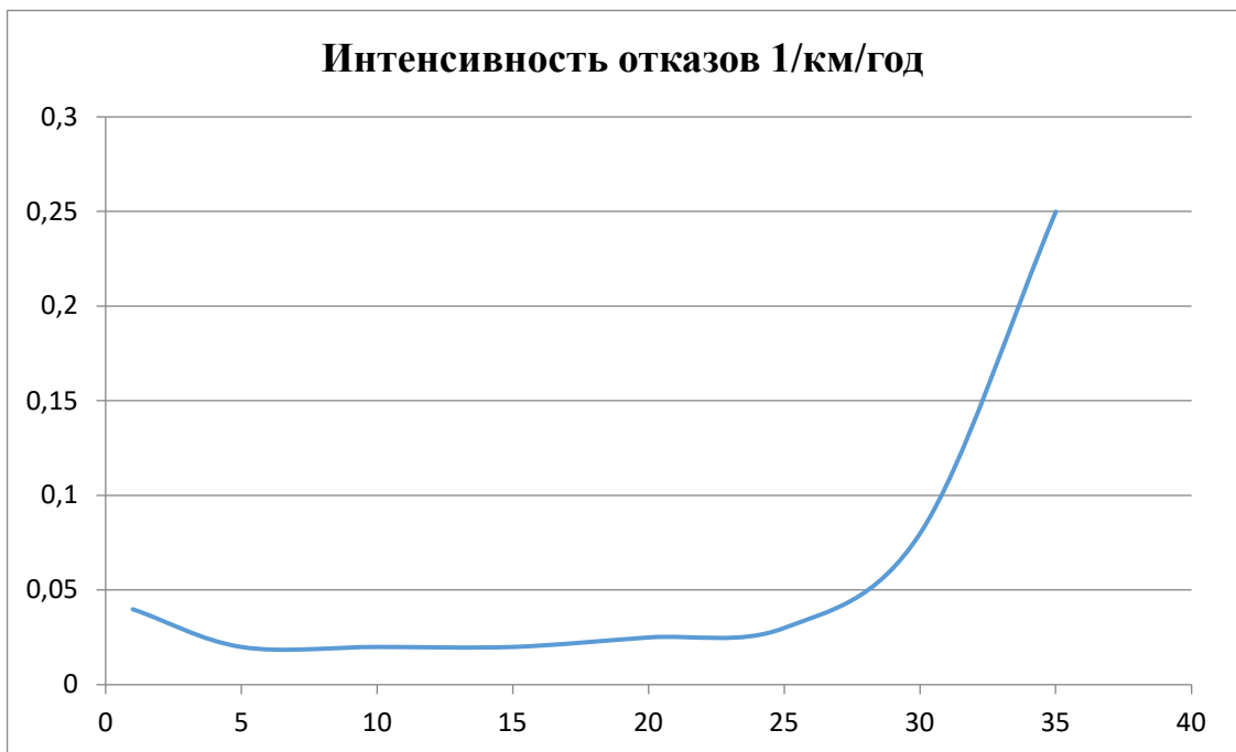
Рисунок 2-1 - Интенсивность отказов
