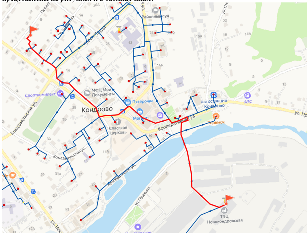
Рисунок 4 - Путь движения теплоносителя от источника тепловой энергии до конечного потребителя, в зоне действия КБК ТЭЦ (направление 2)
