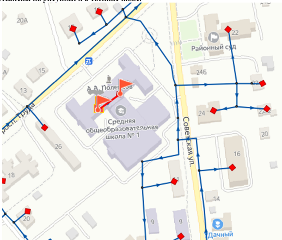
Рисунок 8 - Путь движения теплоносителя от источника тепловой энергии до конечного потребителя, в зоне действия котельной ул. Советская, 13
