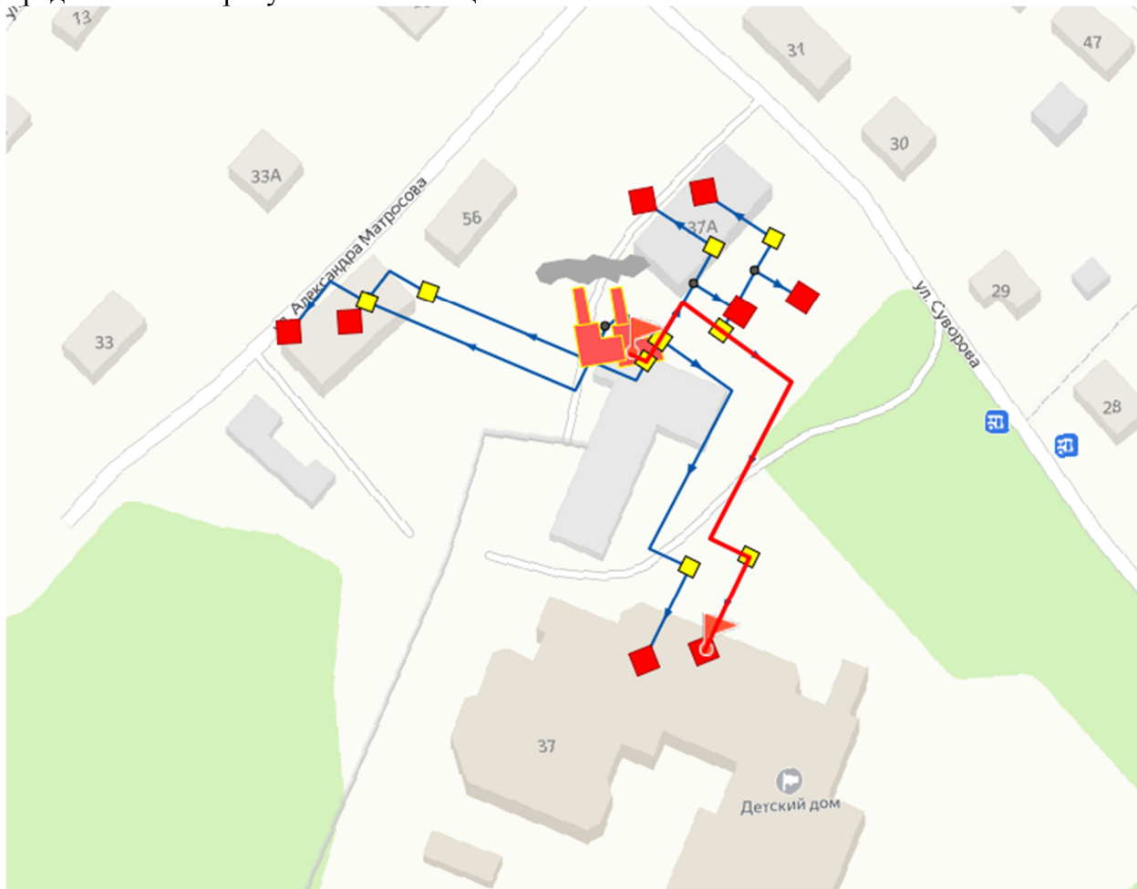
Рисунок 6 - Путь движения теплоносителя от источника тепловой энергии до конечного потребителя, в зоне действия котельной ул. А. Матросова
