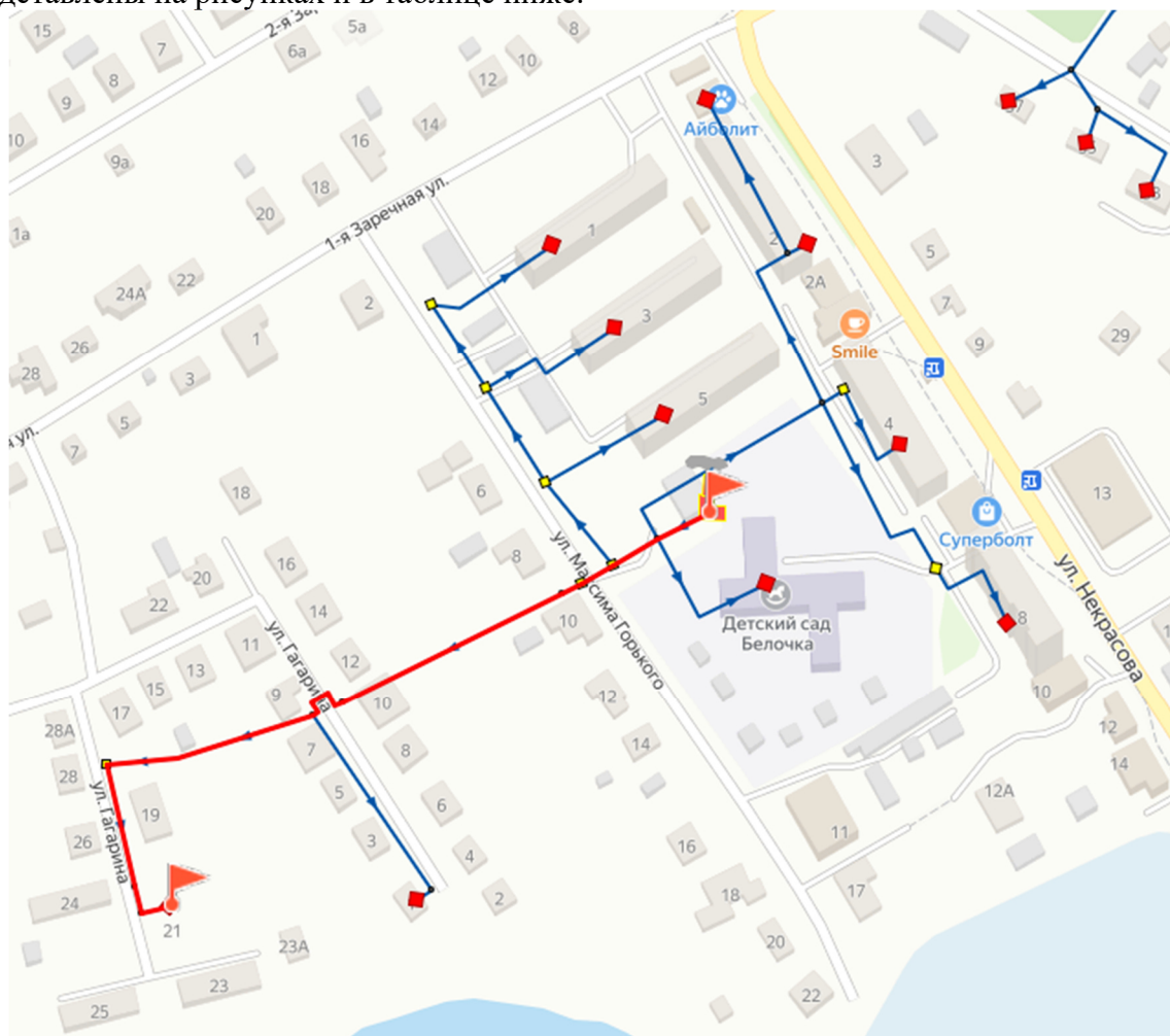
Рисунок 5 - Путь движения теплоносителя от источника тепловой энергии до конечного потребителя, в зоне действия котельной ул. М. Горького
