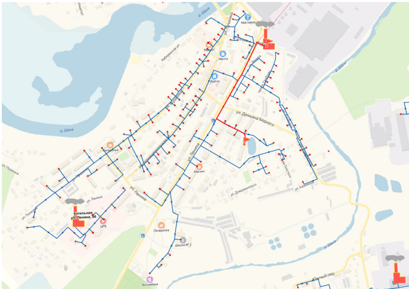
Рисунок 6.4-3 – Путь для построения пьезометрического графика участка от БМК-1 (Юг) до потребителя ул. Дзержинского, 3
